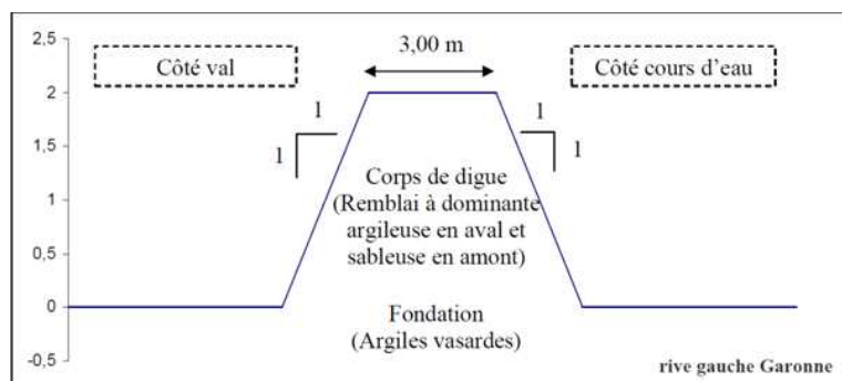
Figure 95 : Profils des digues - Source : SIJALAG – Etude de dangers des ouvrages de protection du SIJALAG- 2015
