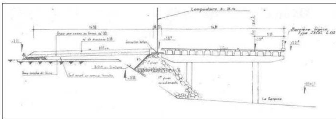
ouvrage de protection contre les inondations en partie aval : remblai routier (type 3)
