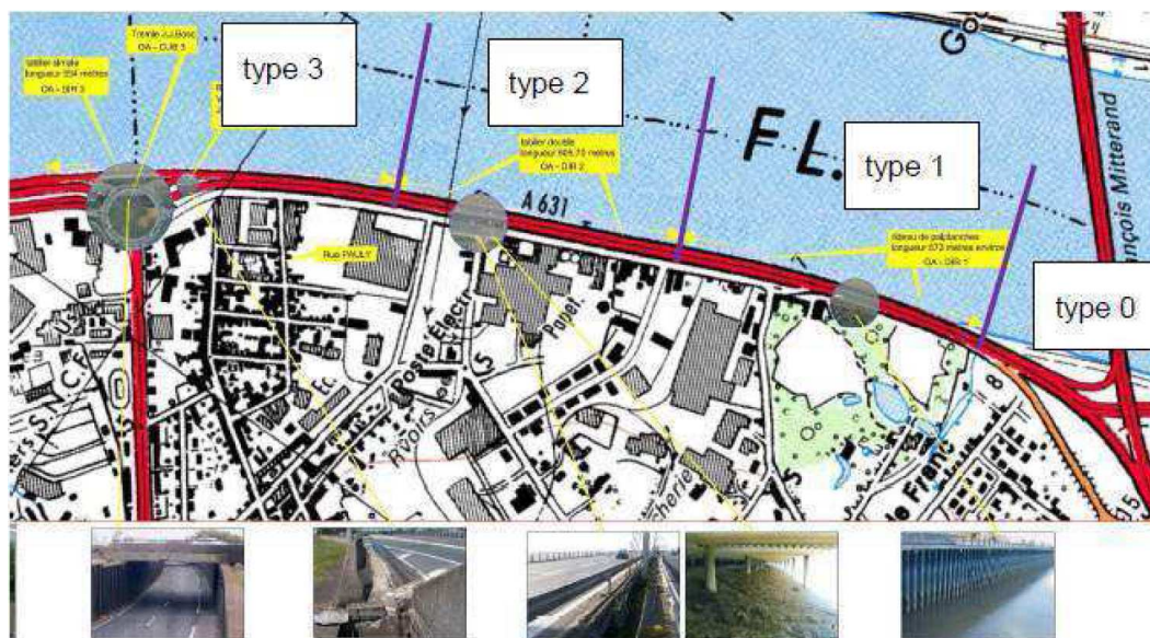
Figure 117 : Typologie de la digue de Saint-Jean Belcier - Source : Bordeaux Métropole – Etude de dangers des digues de Bègles - 2014
