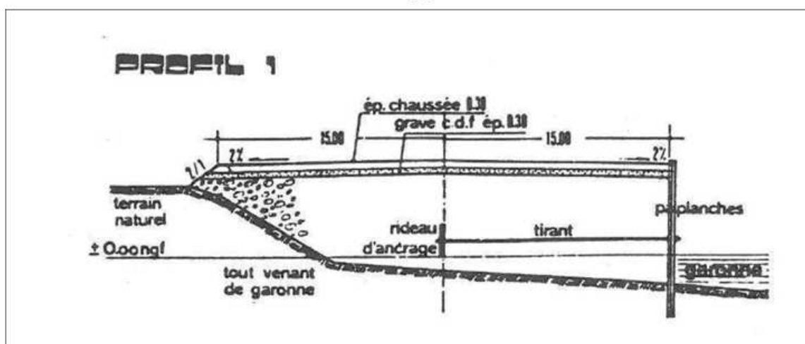
ouvrage de protection contre les inondations en partie amont : palplanches et remblai (type 1)
