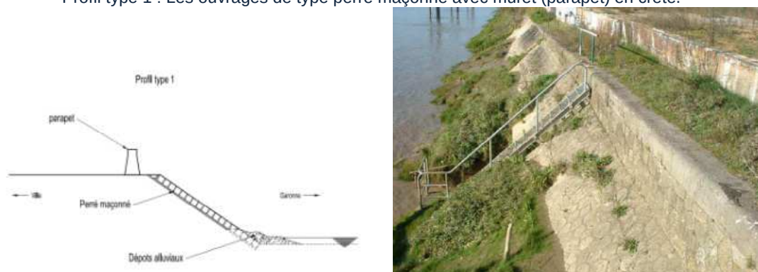
Figure 102 : Dignes de type perré maçonné avec muret en crête - Source : Etude de danger des ouvrages de protection du SPIRD – 2013
