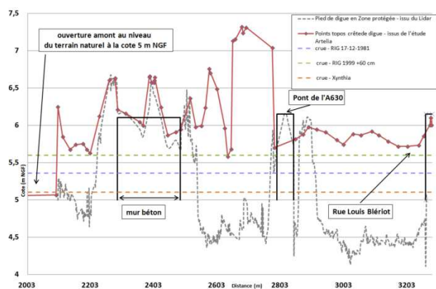
Figure 128 : Profil en long de la digue en rive gauche de l'Estey de Franc - Etude de dangers des digues non classées de Bègles – 2014
