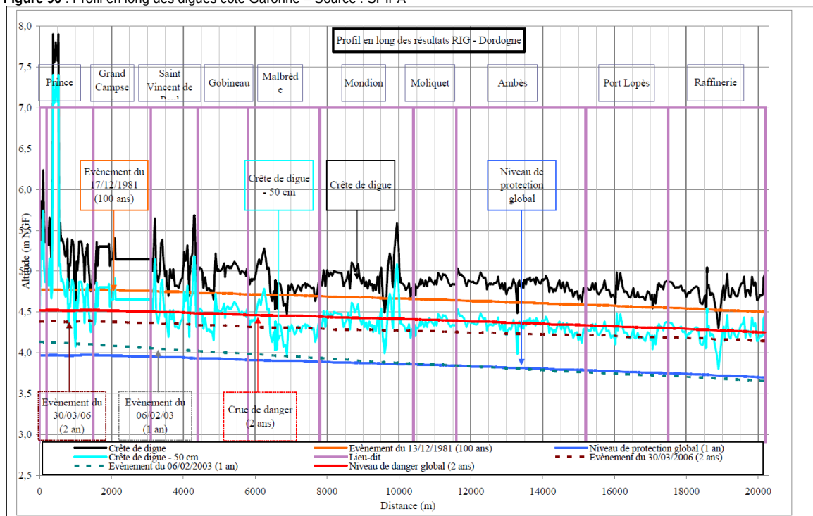
Figure 91 : profil en long des digues coté Dordogne – Source : SPIPA
