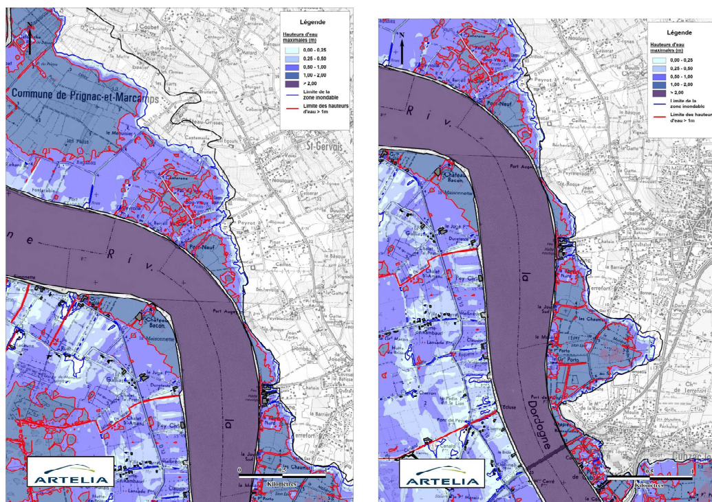
Figure 155 : Analyse du comportement hydraulique du secteur de Saint-André-de-Cubzac - Source : SMIDDEST - Etude préliminaire de définition des mesures de protection à mettre en place sur 14 sites riverains de l'Estuaire de la Gironde pour en réduire la vulnérabilité au tire de l'événement de référence – 2015
