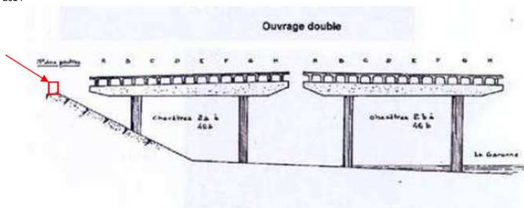
Ouvrage de protection contre les inondations en partie centrale : muret (type 2)
