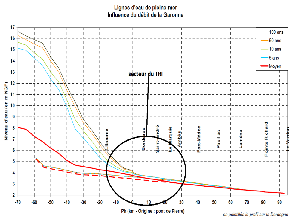
Figure 29 : Lignes d'eau de plein-mer - Influence du débit de la Garonne - Source : SMIDDEST - Referentiel Inondation Gironde, rapport d'étude 4
