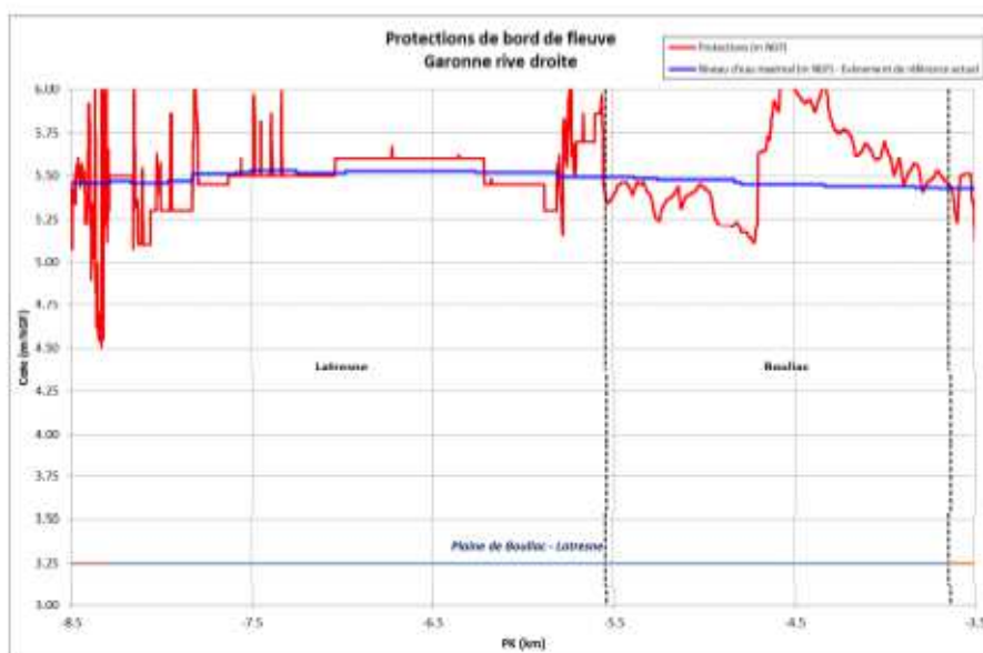
Figure 143 : Profil en long des digues du casier hydraulique Bouliac-Lastresne – Source : DDTM33 – Révision du PPRL de l'agglomération bordelaise – 2014
