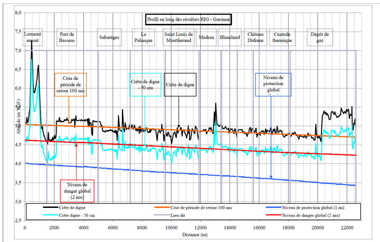
Figure 90 : Profil en long des digues coté Garonne – Source : SPIPA
