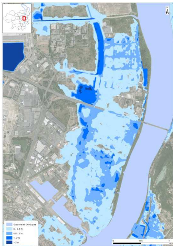
Figure 100 : Hauteurs d'eau - configuration digues actuelles (sans défaillance) - Source : DDTM33 - Révision du PPRI de l'agglomération bordelaise – 2014
