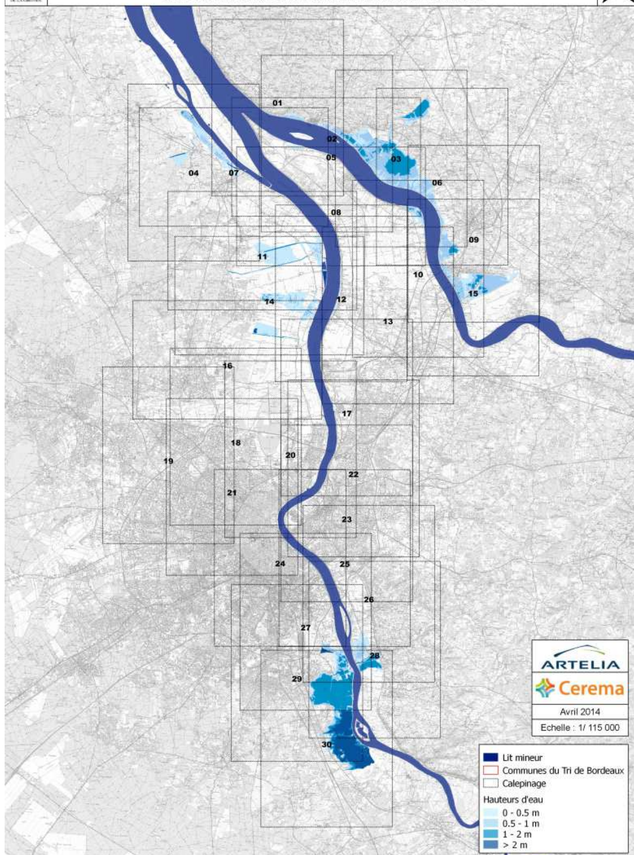
Figure 14: Carte des surfaces inondables - type : débordement fluvial – Evenement moyen - Source : DDTM 33 – Rapport d'accompagnement des cartographies du TRI Bordeaux - décembre 2014
