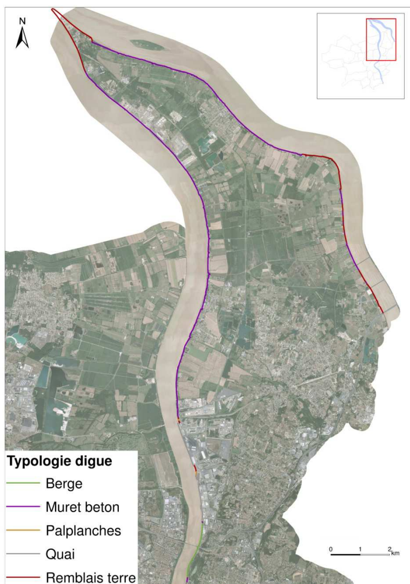
Figure 88 : Typologie des digues de la Presqu'île d'Ambès - Source : Bordeaux Métropole - 2016
