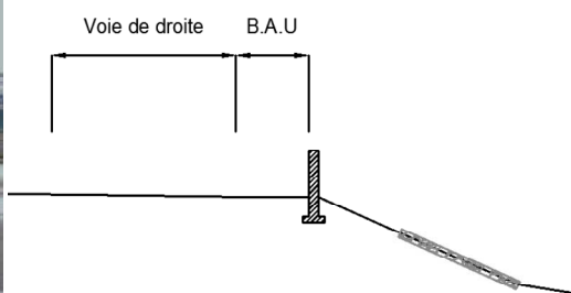
Figure 111 : Digue de type mur - ouvrage de Saint-Jean-Belcier : Source : EPA - Etude de danger de la digue Saint-Jean Belcier - 2013
