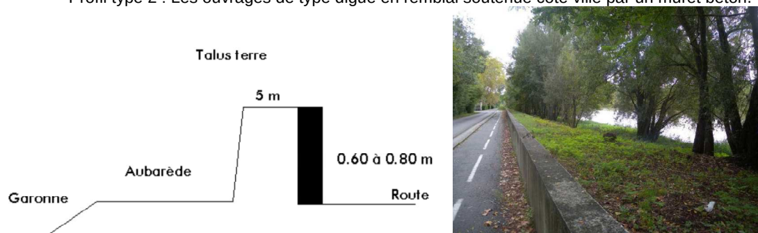
Figure 103 : Dignes en remblais - - Source : Etude de danger des ouvrages de protection du SPIRD - 2013
