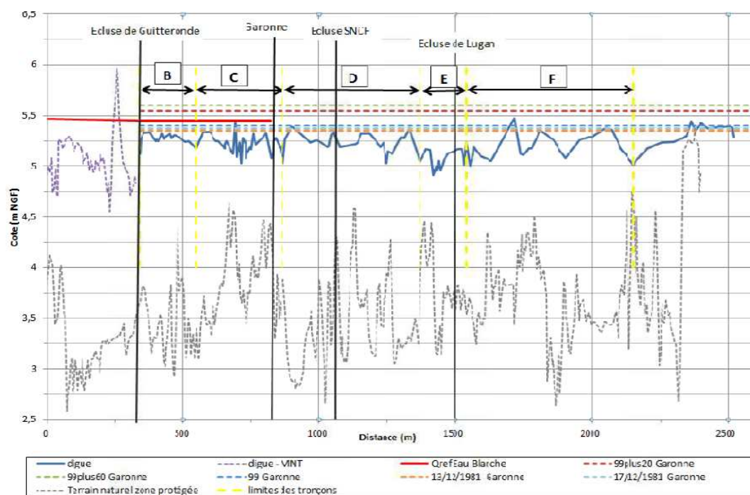
Figure 135 : Profil en long de la digue classée de villenave d'Ornon en bord de Garonne - Source : Bordeaux Metropole - Etude de dangers des digues classées de PLABO S.A.S – 2014
