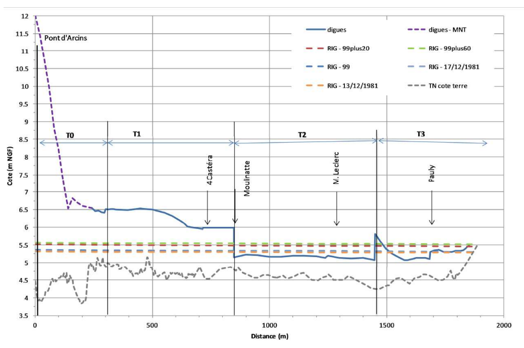
Figure 122 : Profil en long des digues de Bègles - Source : Etude de dangers des digues de Bègles - 2014
