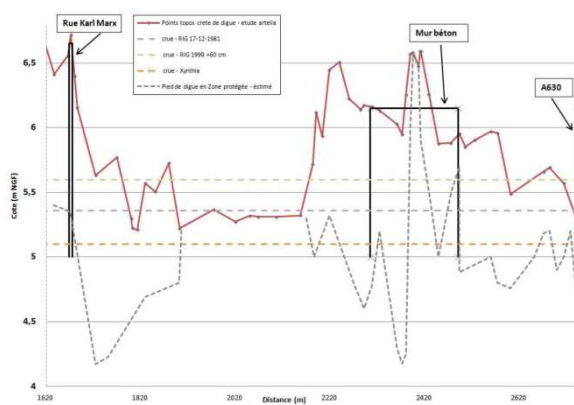
Figure 129 : Profil en long de la digue en rive droite de l'Estey de Franc - Etude de dangers des digues non classées de Bègles – 2014
