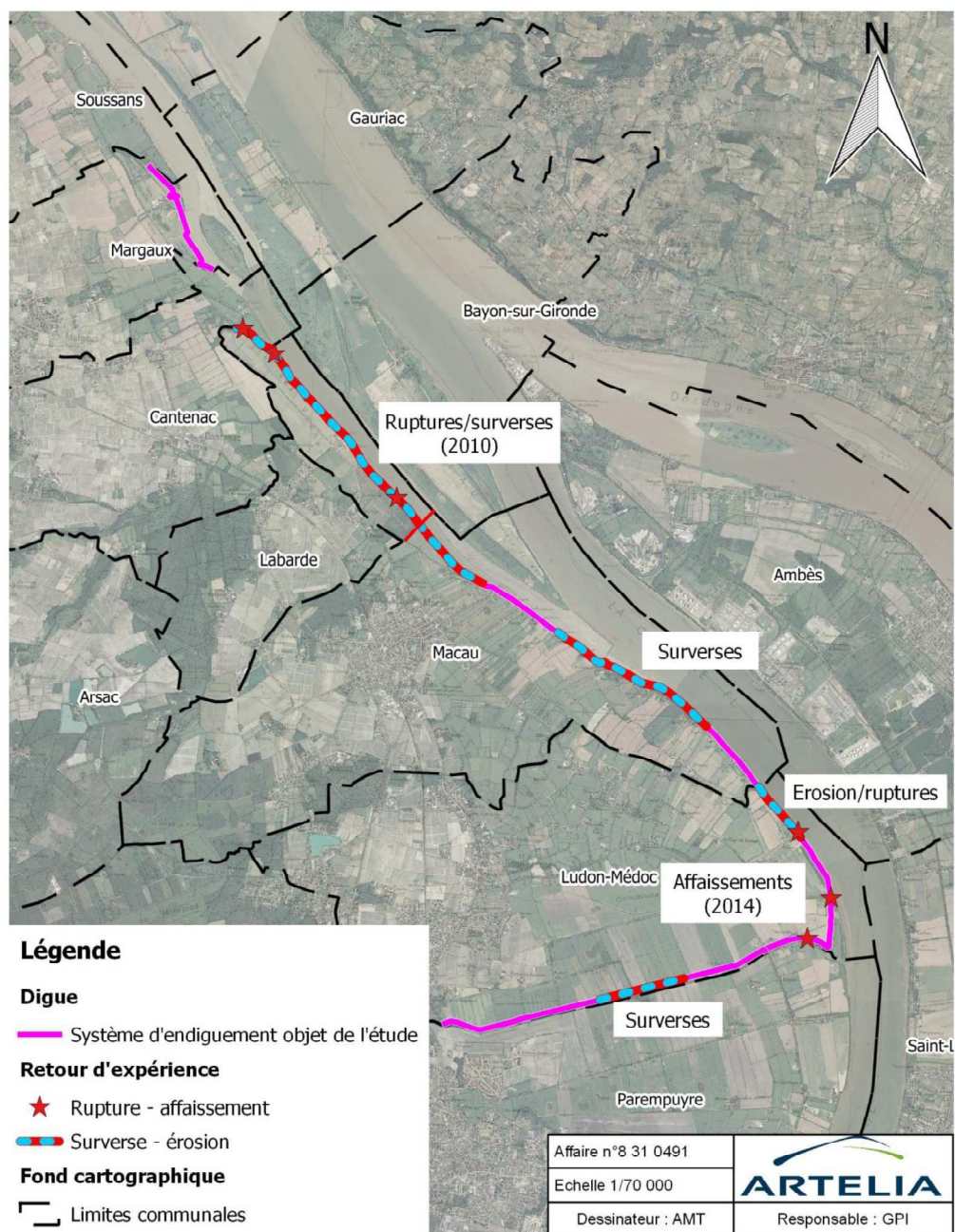
Figure 148 : Retour d'expérience des défaillances réelles des ouvrages de protection du SMBVAM - Source : SMBVAM - Etude de dangers des ouvrages de protection contre les inondations sur les communes de Ludon Medoc, Macau, Labarde, Cantenac et Margaux – 2016
