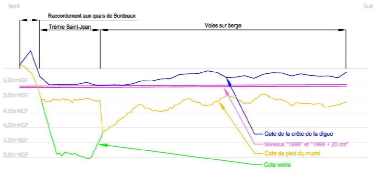
Figure 113 : Profil en long des digues de Saint-Jean Belcier – Source : EPA
