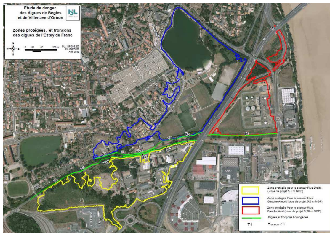
Figure 131 : Zone protégée par les digues de l'Estey de France à Bègles- Source : Bordeaux Métropole - Etude de dangers des digues non classées de Bègles – 2014
