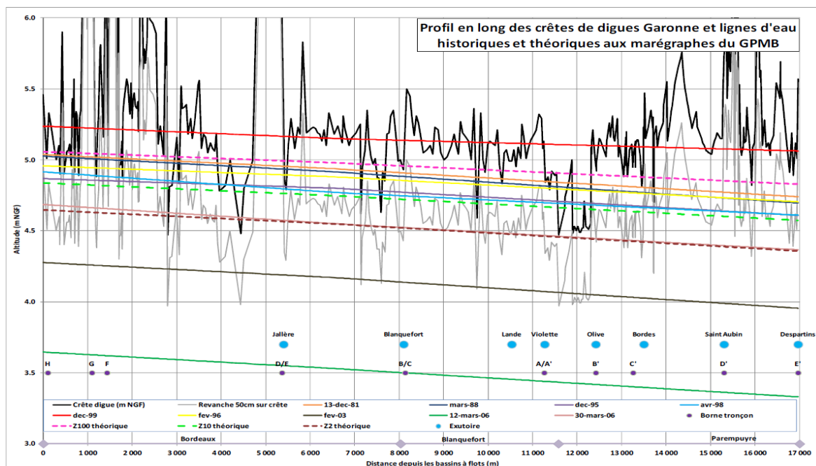
Figure 33. Ligne d'eau par événement fluvio-maritime (source RIG)
