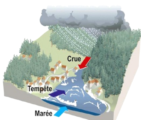
Figure 28 : Schéma de la formation d'une inondation fluvio-maritime –Source : Bordeaux Metropole
