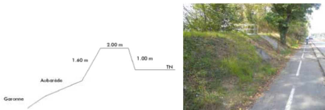
Figure 105 : Dignes en remblai non revêtue - - Source : Etude de danger des ouvrages de protection du SPIRD – 2013
