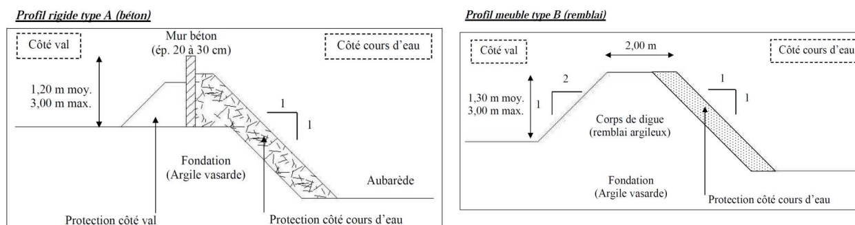
Figure 87 : Profils des digues - Source : SPIPA – Etude de dangers des ouvrages de protection du SPIPA – 2015
