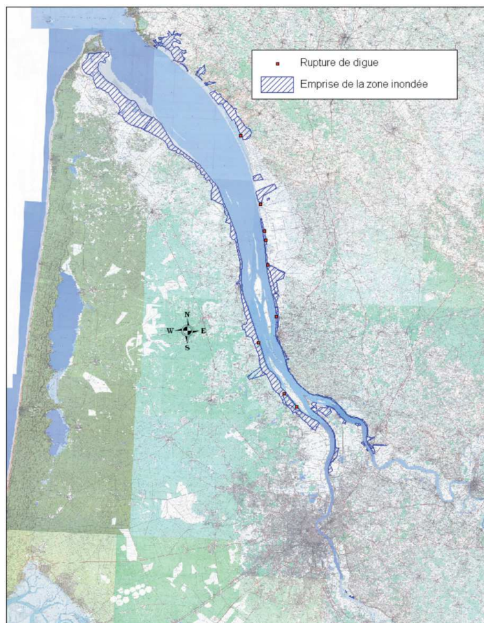
Figure 39 : Emprise de la zone inondée constatée lors de la Tempête Xynthia – Source : SMIDDEST
