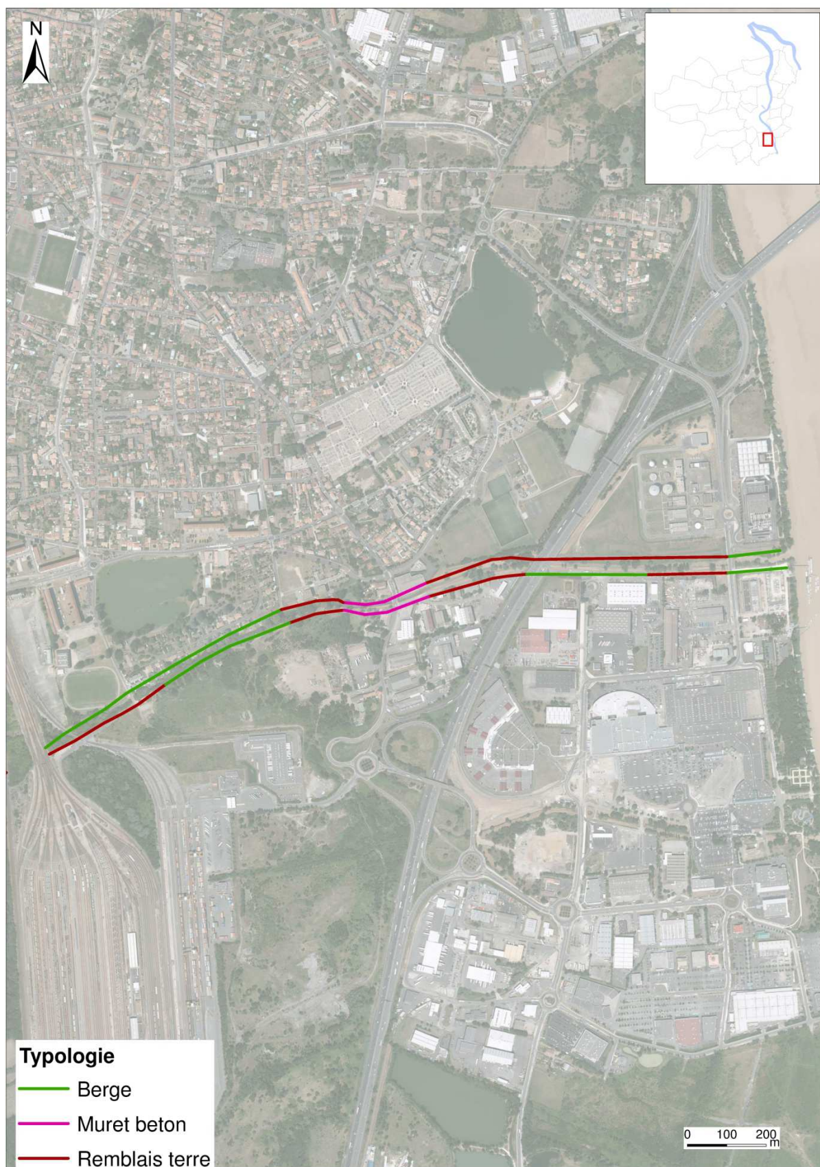
Figure 130 : Typologie des digues de Bègles - Source : Bordeaux Métropole - 2016
