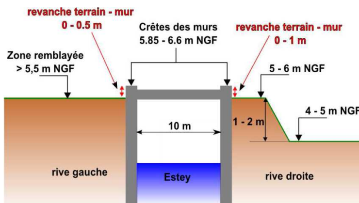
Figure 127 : Coupe schématique du linéaire comportant le mur béton - Source : Bordeaux Métropole - Etude de dangers des digues non classées de Bègles – 2014
