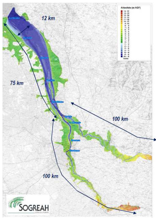
Figure 31 : Influence de la marée - Source : SMIDDEST- RIG phase 1
