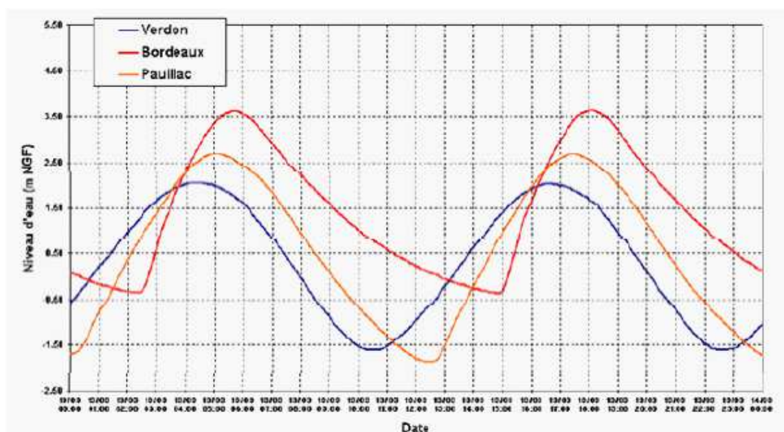
Figure 32 : Asymétrie de l'onde de marée – Source : SMIDDEST – RIG Phase 1
