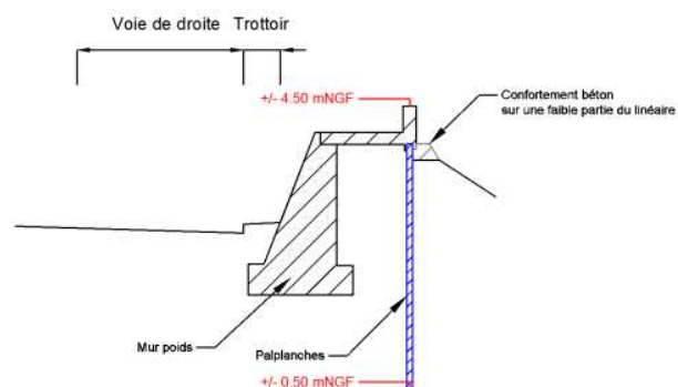
Figure 110 : Digue de type rideau palplanches - ouvrage de Saint-Jean-Belcier : Source : EPA - Etude de danger de la digue Saint-Jean Belcier - 2013
