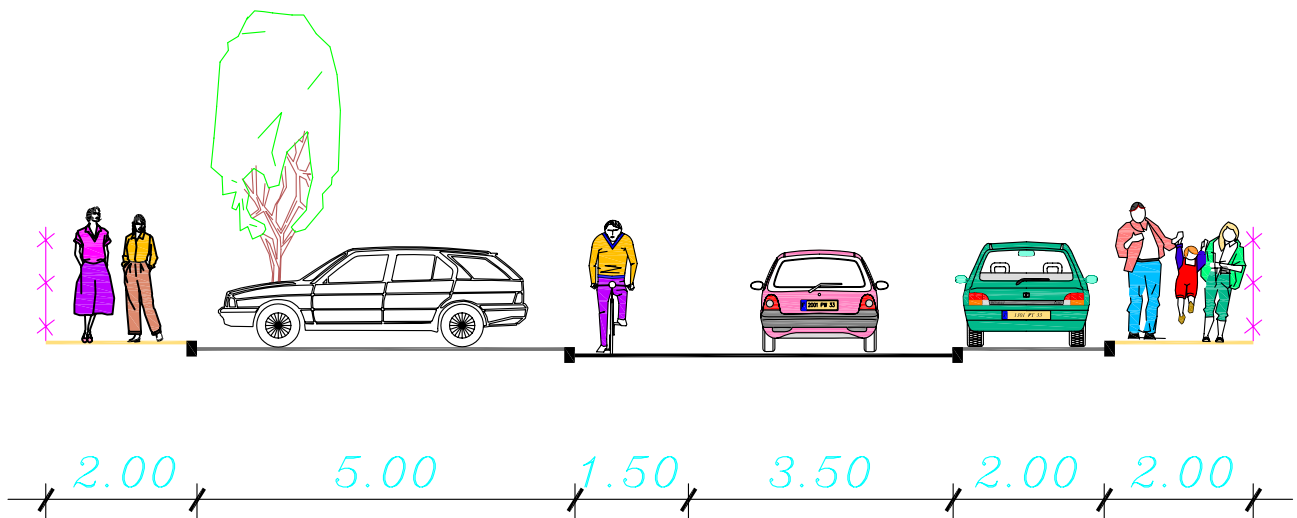
Profil en travers type futur
