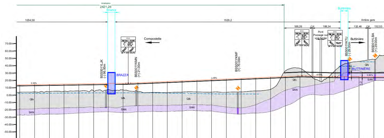
Figure 121 : Extrait du profil en long du tracé entre Brazza et Buttinière
