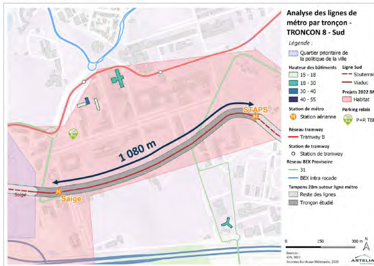
Figure 31. Zoom sur le tronçon 8 : STAPS – Saïge
