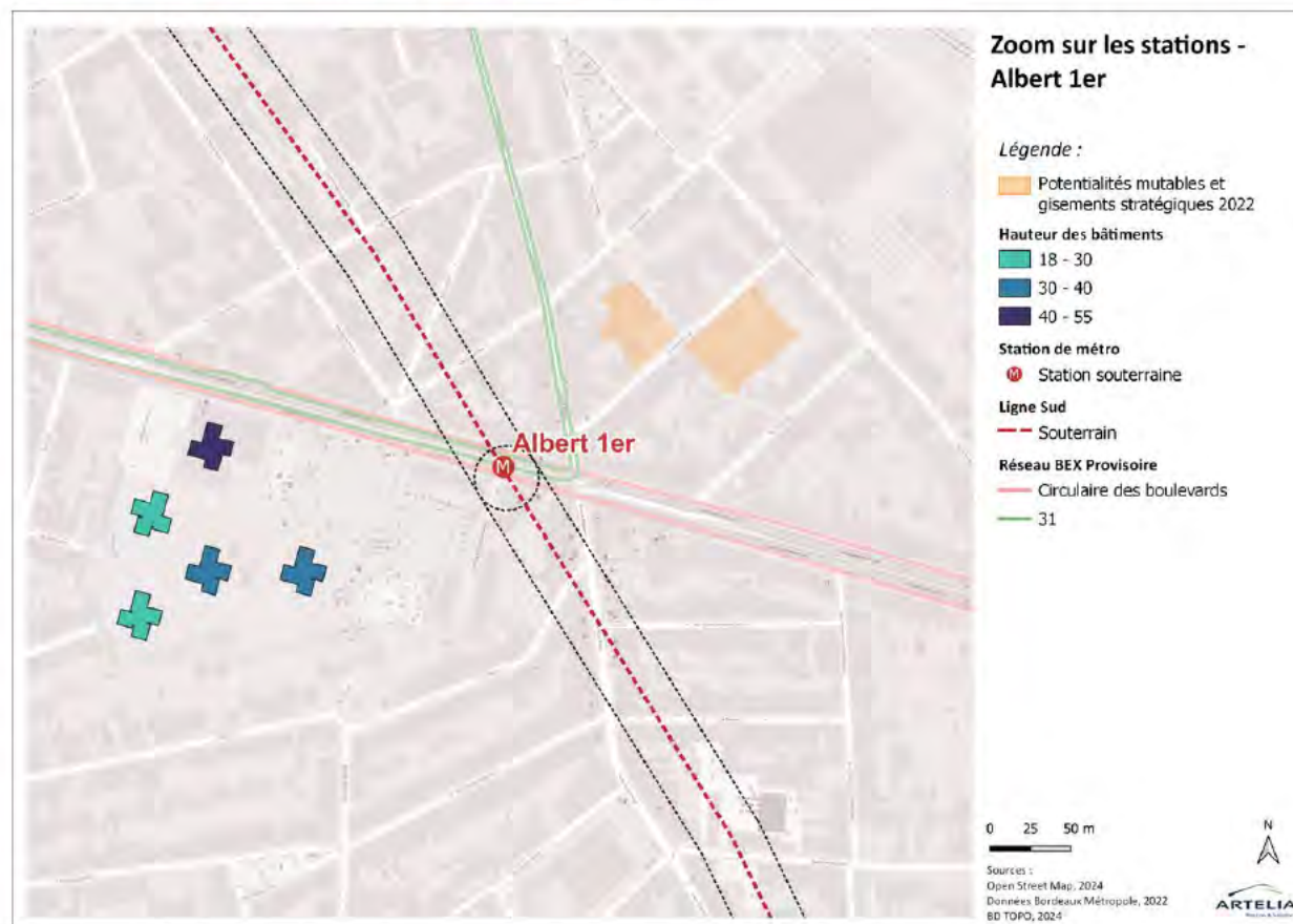
Figure 54. Zoom sur la station 11 : Albert I er
